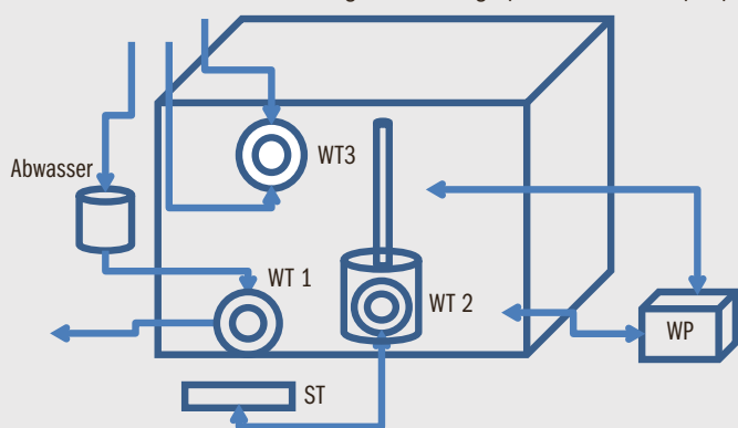
Seitlich und oben gedämmter Betonspeicher mit 23 m 3 Wasser gefüllt als Energiequelle für die Wärmepumpe
